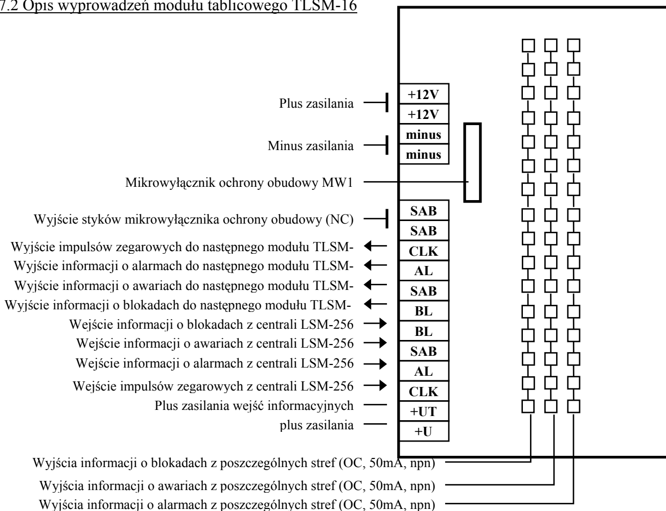
Rys. 9 Opis wyprowadzeń modułu tablicowego TLISM-16
