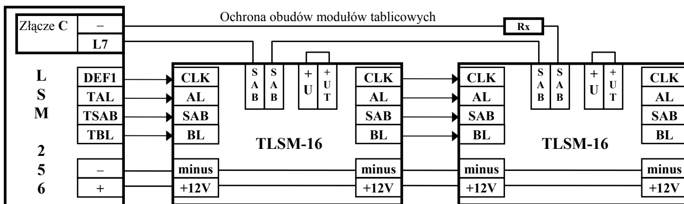
Rys. 10 Podłączenie modułów tablicowych TLISM - 16 do centrali LSM-256.
