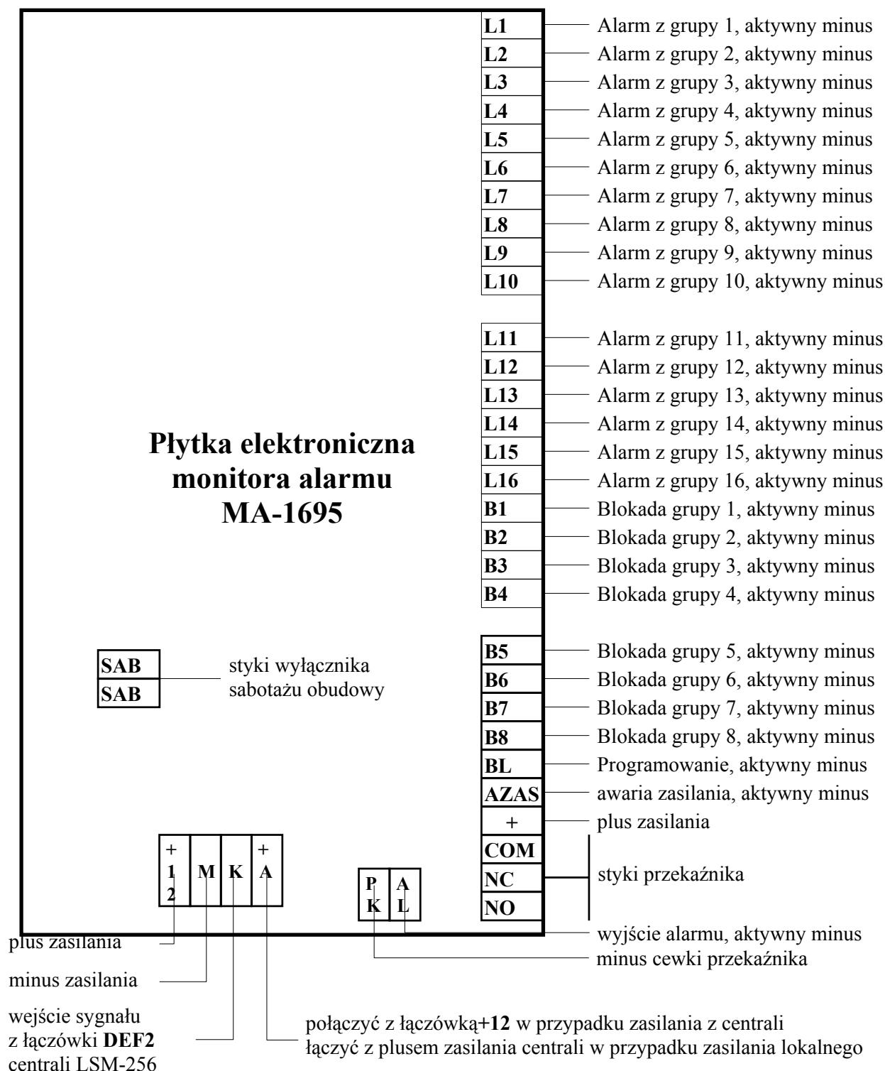
Rys. 12. Opis wyprowadzeń na płytce moduły MA-1695
